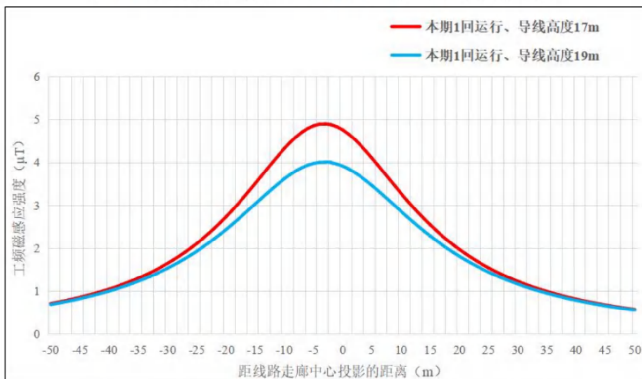
图 3-6 本项目架空线路下距地面 1.5m 处工频磁感应强度预测曲线图
