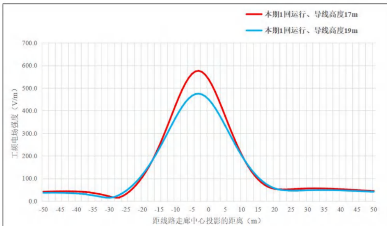
图 3-5 本项目架空线路下距地面 1.5m 处工频电场强度预测曲线图
